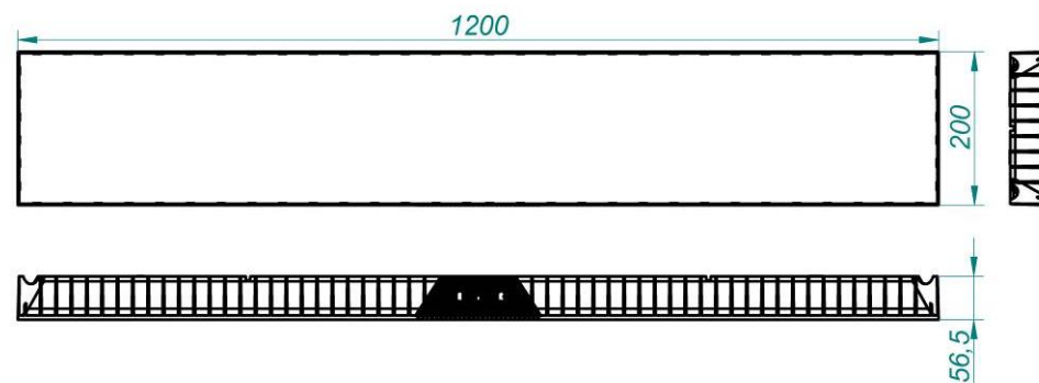
Рисунок 1б Светильник «L-school 32», «L-school 55»
