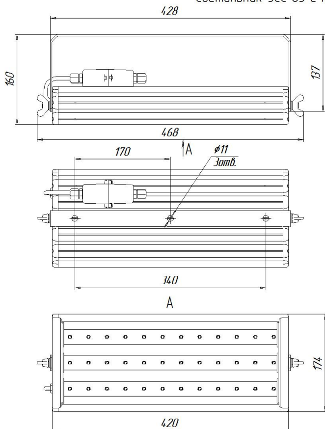
Светильник УСС 65 с креплением скоба
