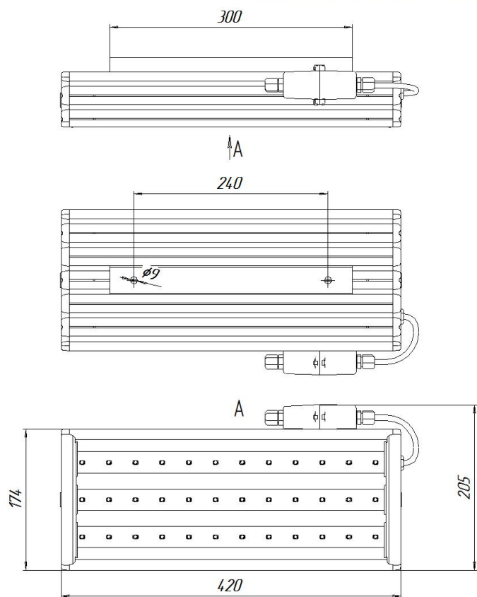
Светильник УСС 65 потолочное крепление
