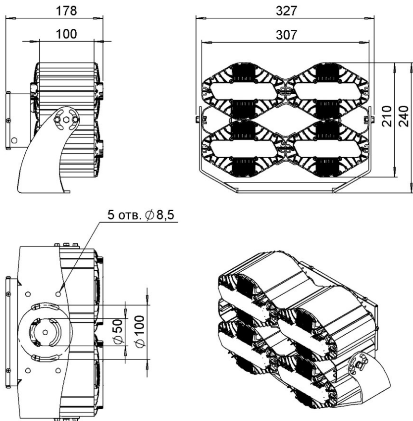
Рисунок 2 Светильник «L-lego 220» Поворотное крепление.
