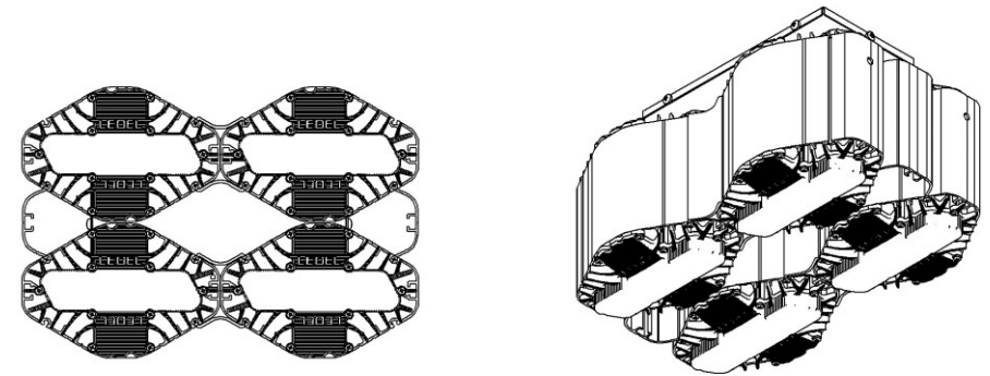
Рисунок 1 Светильник «L-lego 220» Подвесное крепление.
