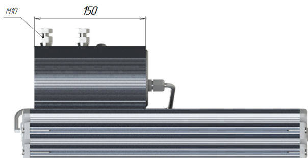
Светильник УСС-65 Магистраль Ш1-2; с креплением на консоли
