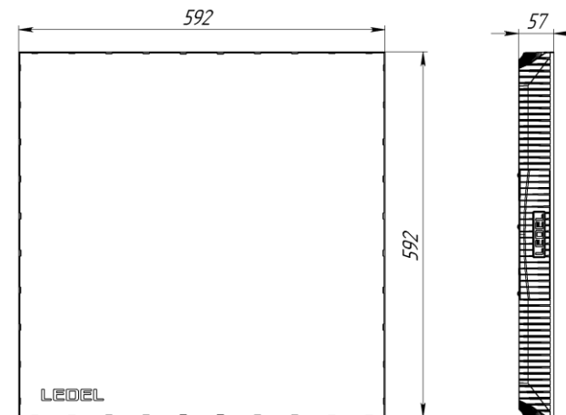
Рисунок 1 Светильник «L-office 55/Em»
