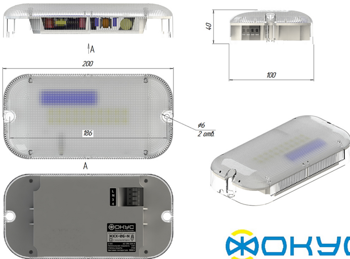
Светодиодный светильник ЖКХ-06; с аккумулятором
