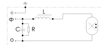
Рисунок 5 – Схема подключения к сети светильников ПКУ15
