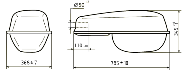
Рисунок 1 – Светильники серии ЖКУ15/ПКУ15/ГКУ15...101/105/107
