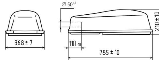
Рисунок 3 - Светильники серии ЖКУ15/ПКУ15/ГКУ15...103
