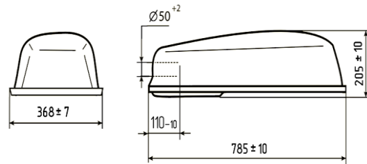
Рисунок 2 – Светильники серии ЖКУ15/ПКУ15/ГКУ15...102
