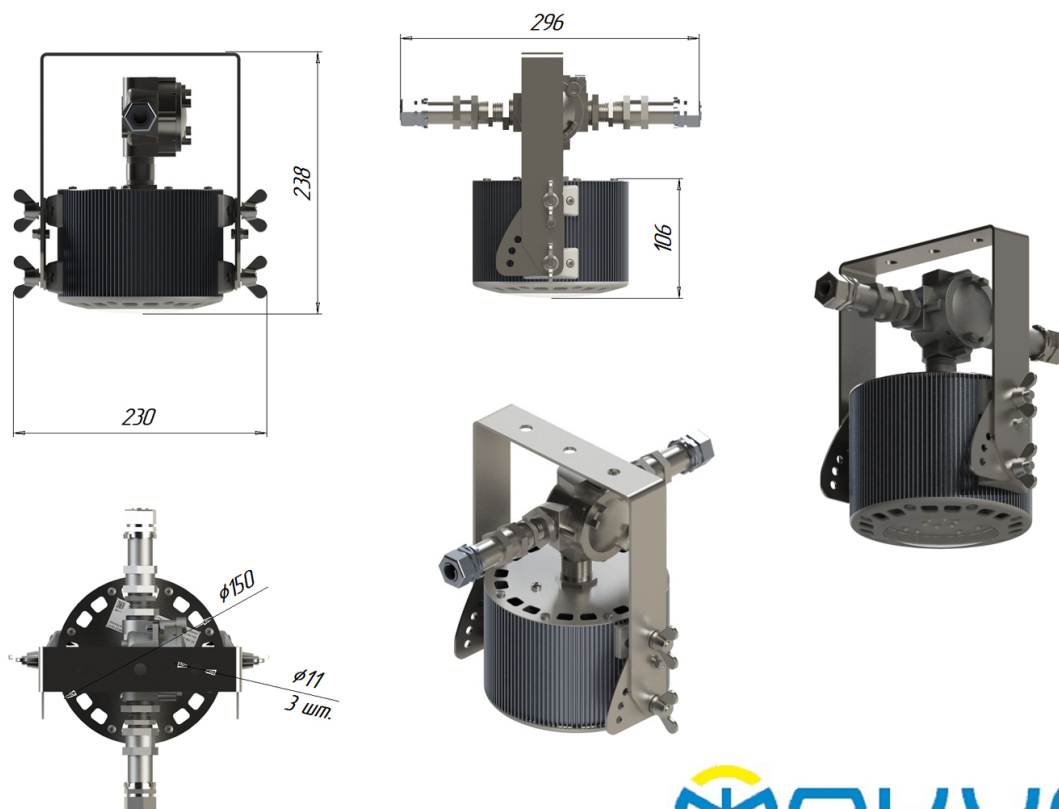
Светильник ПСС-15 ПКК с 1Ех маркировкой крепление на скобе
