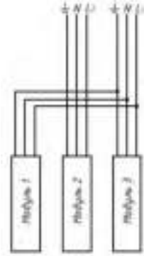
Вариант подключения №2. Подключение помодульно.
