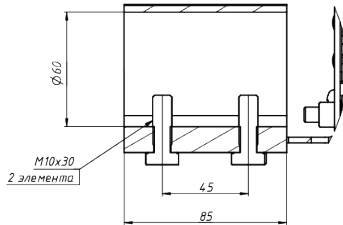
Вид - А
