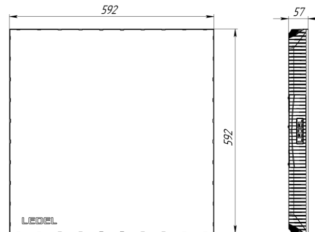
Рисунок 1 Светильник «L-office 32/Em»
