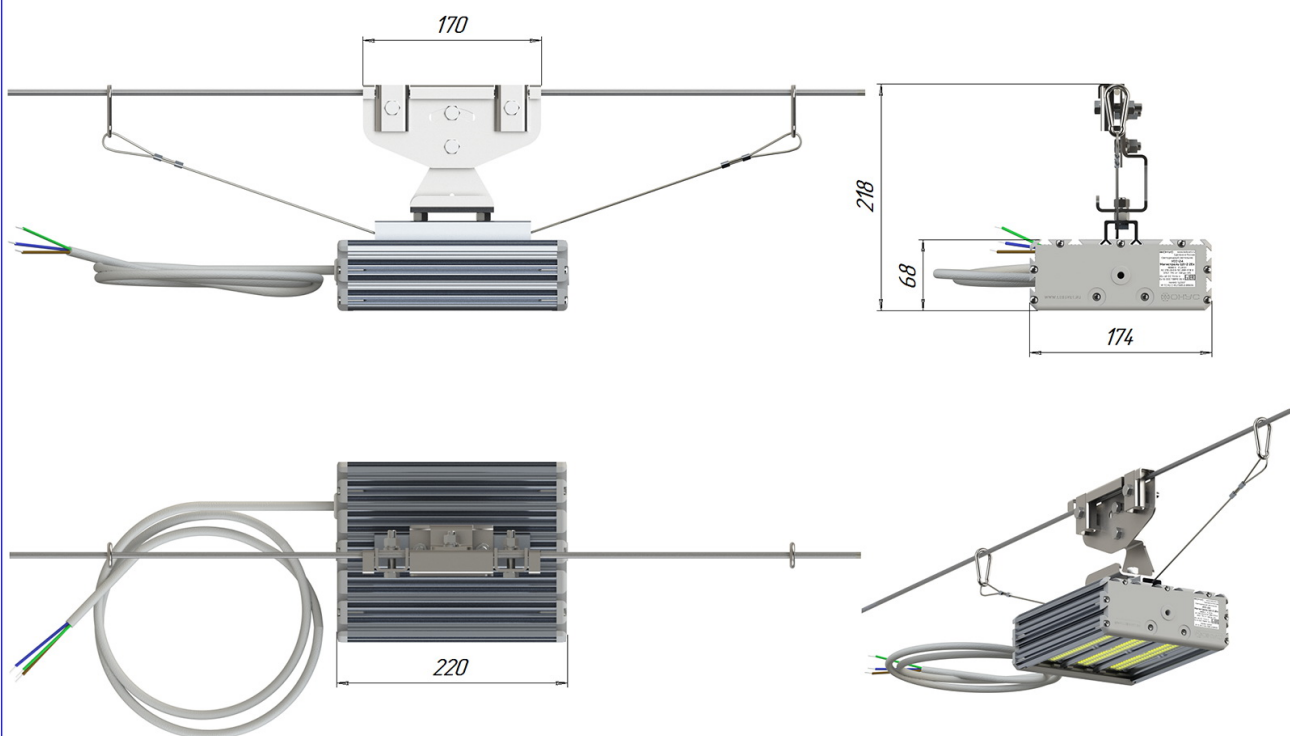
Светильник УСС-24 Магистраль Ш1-2 2Ех; с креплением на трос
