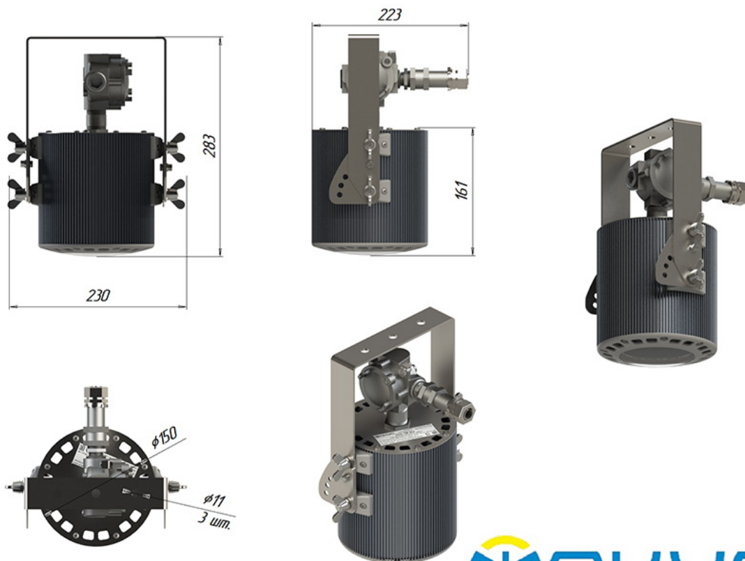
Светильник ПСС-50 с 1Ех маркировкой крепление на скобе
