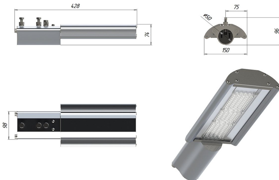
Светильник УСС-50 Катана Трасса ШБ-1; консольное крепление
