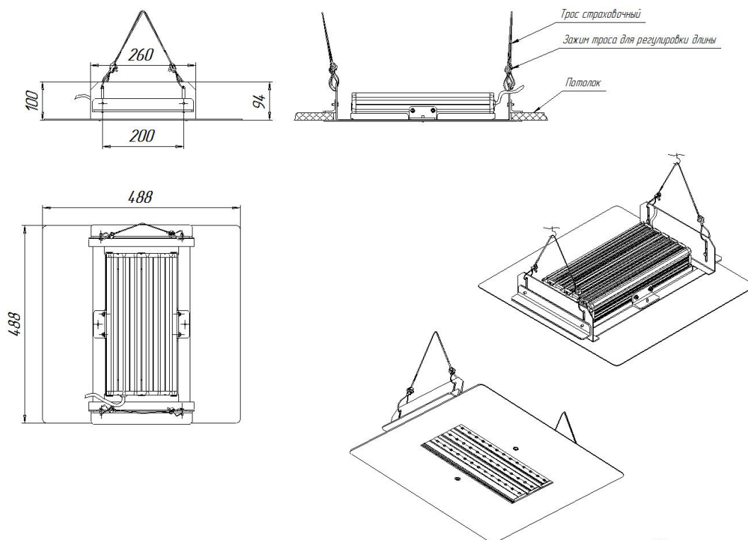
Светильник УСС 42 АЗС с 2Ех маркировкой; рамочное крепление
