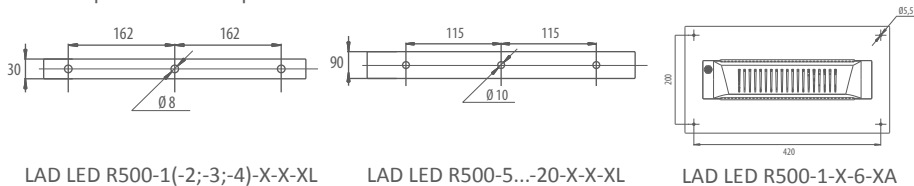
Рис. 1. Крепежные отверстия
