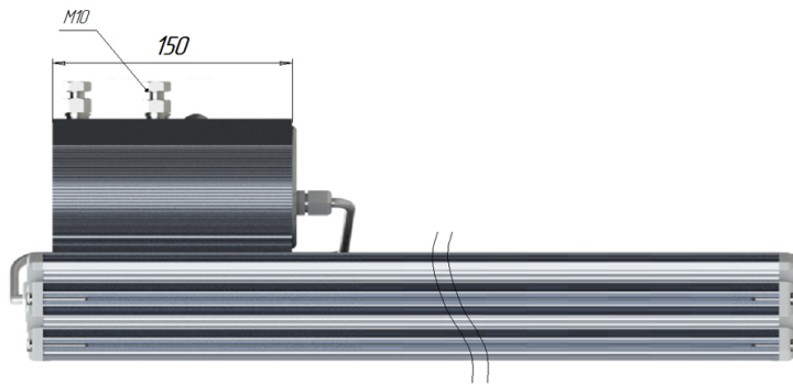
Светильник УСС-180 Магистраль Ш1-2; с креплением на консоли
