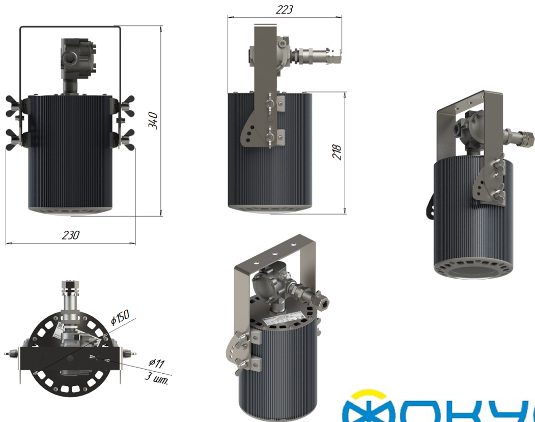
Светильник ПСС-70 с 1Ex маркировкой крепление на скобе
